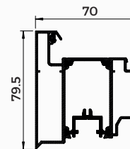
WQ41 DOOR 'T' SASH
