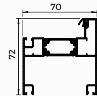
WQ03 DEEP OUTER FRAME
