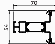
WQ12 SLIM 'T' MULLION
